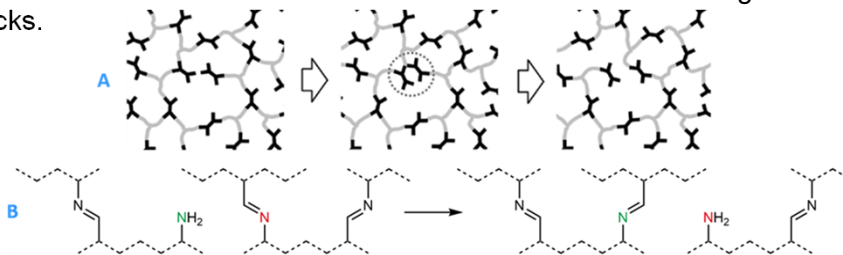
Abbildung 1: Schematische Darstellung des Bindungsaustauschs in einem Netzwerk (A); Bindungsaustausch zwischen Aminen und Imin (B).
